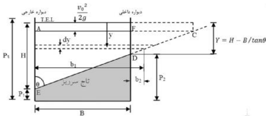
شکل ۵- پروفیل عرضی تاج سرریز شیبدار در پیچ یک آبراهه
