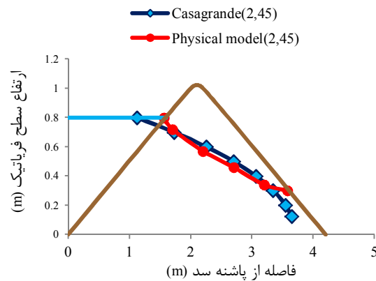
شکل ۱۲- مقایسه خط فریاتیگ در مدل فیزیکی با روش کاساگراند در حالت p/h=2 با زاویه ۴۵ درجه
