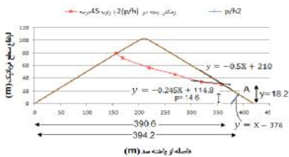
خ) خط نشت زهکش ۲ (p/h) با زاویه ۴۵
