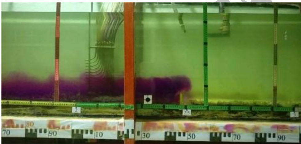
شکل ۱۰- نمایی از برخورد پیشانی جریان غلیظ با موانع
